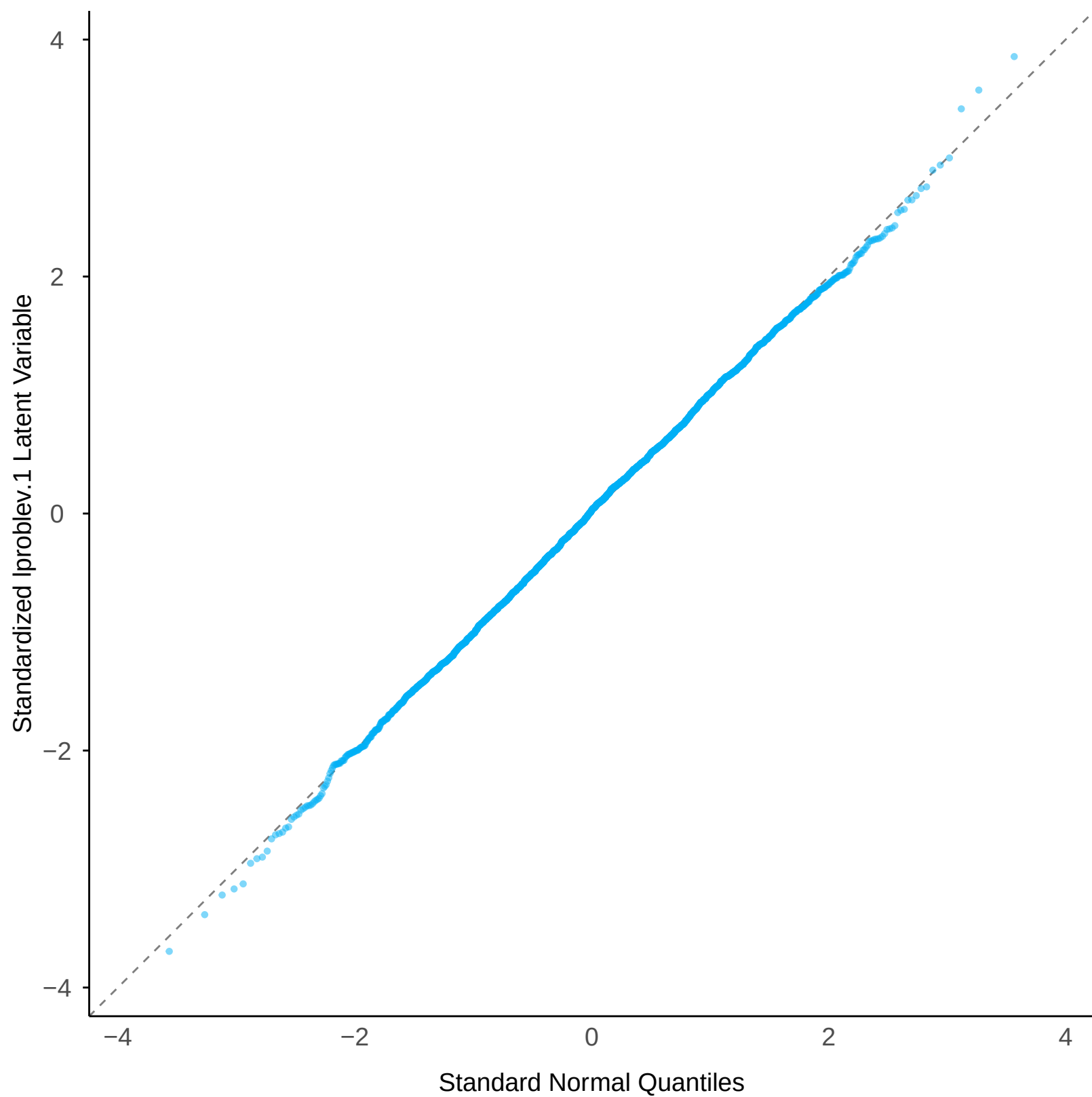
Normal Q-Q: lproblev.1 Latent Variable
