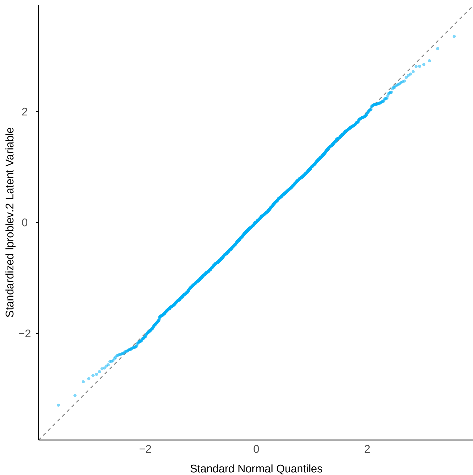
Normal Q-Q: lproblev.2 Latent Variable
